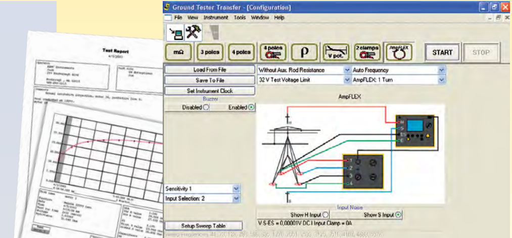
Parametrieren des ausgewählten Messverfahrens und grafische Anzeige des Schaltbilds.
