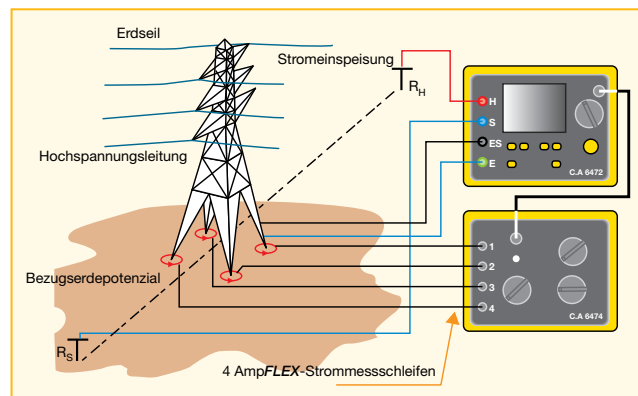
Messung einer Masterdung mit den C.A 6472 + C.A 6474
