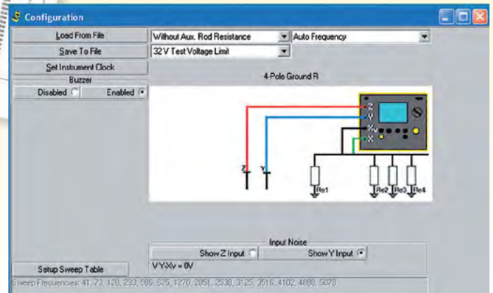
Parametrieren des ausgewählten Messverfahrens und grafische Anzeige des Schaltbilds.
